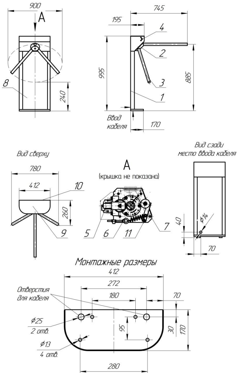
Габаритные и установочные размеры турникета «Ростов-Дон Т83М1»
